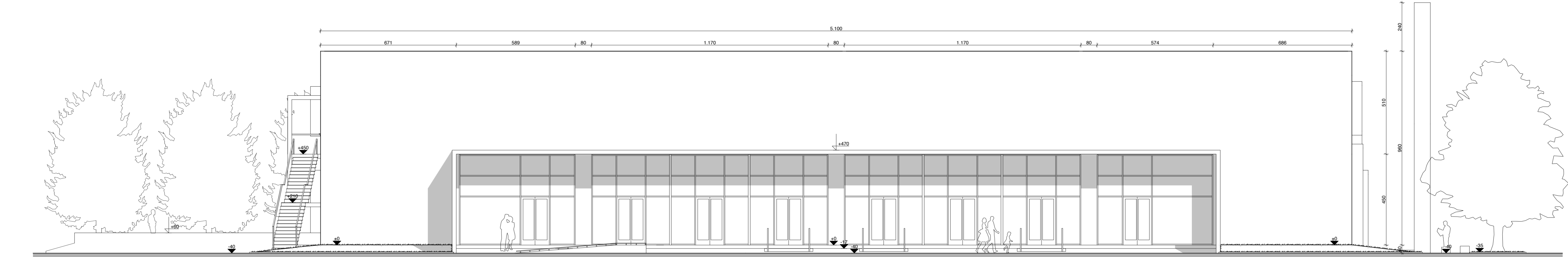
Pros-Ovest 1 : 100
