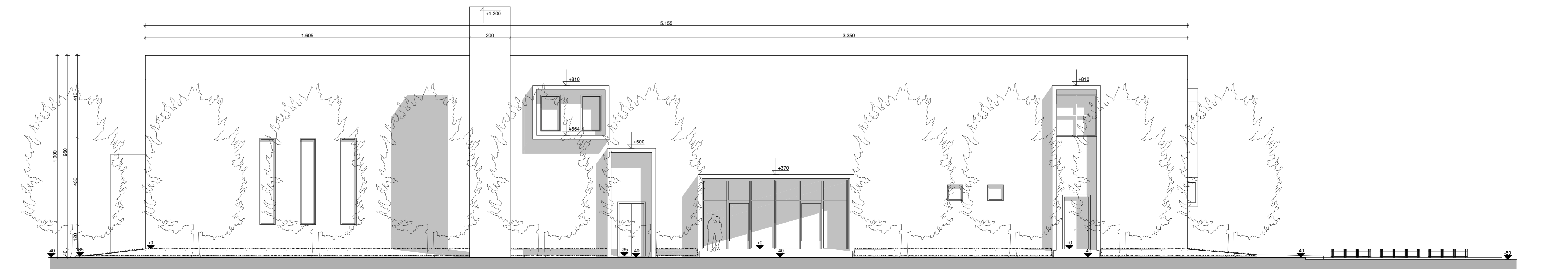
Pros-Sud 1 : 100
