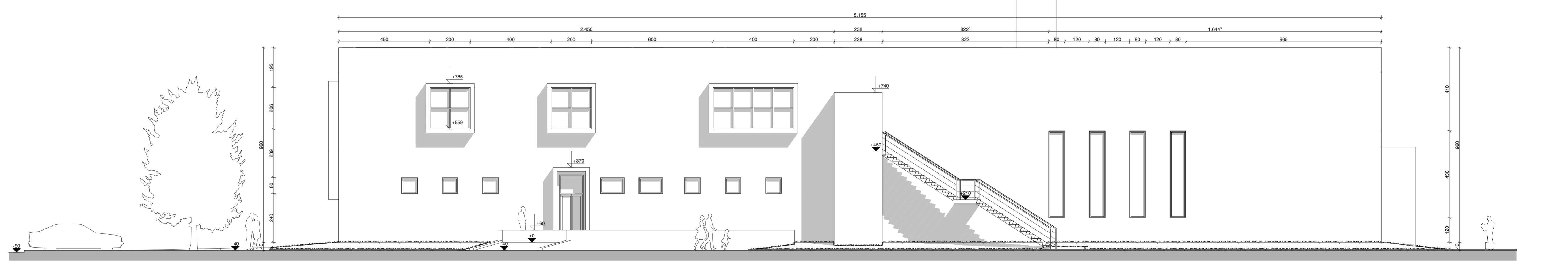
Pros-Est 1 : 100
